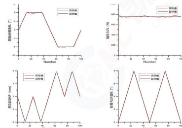
肩关节测试曲线
