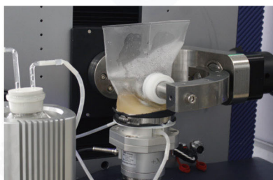
膝关节循环水浴环境
