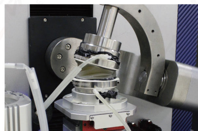
髋关节循环水浴环境
