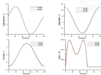
髋关节测试曲线
