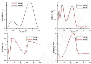
膝关节测试曲线
