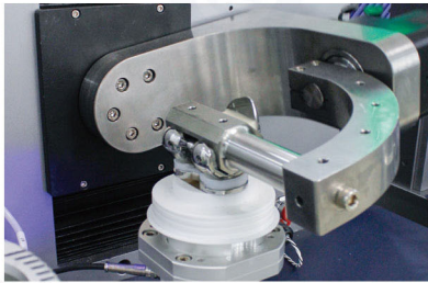
膝关节假体磨损测试
