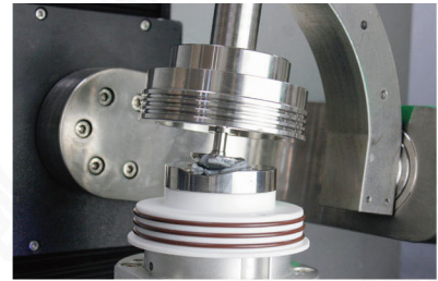
肩关节假体磨损测试
